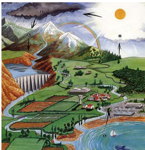
Obr. 3. – koloběh vody v přírodě
