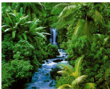
Obr. 3. – deštný prales
